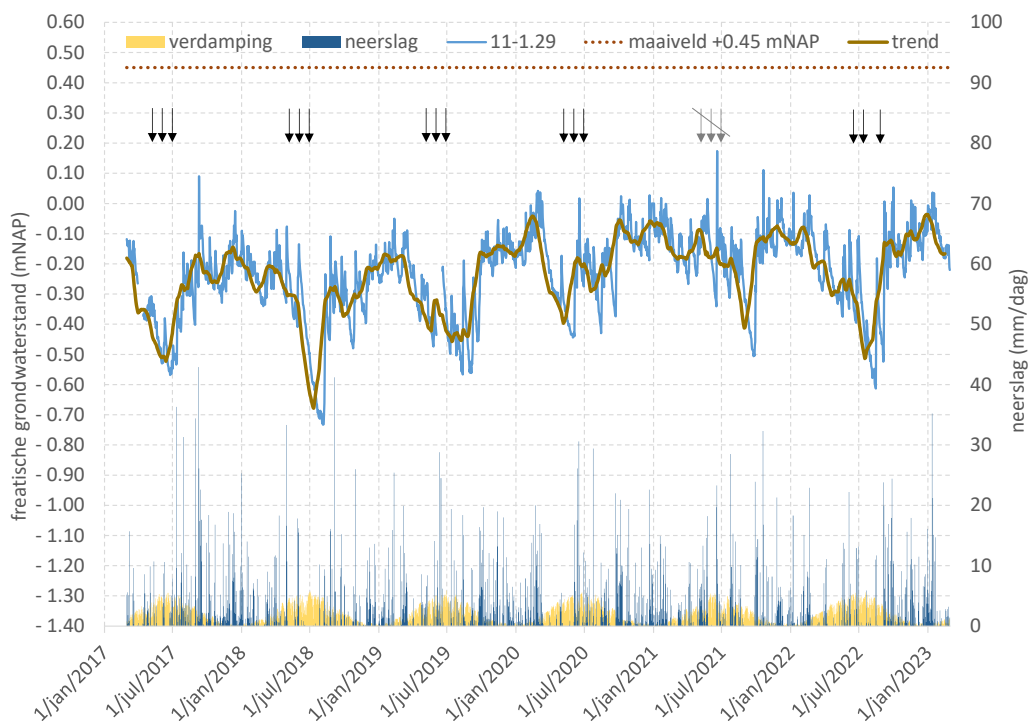
Figuur 23 Freatische grondwaterstanden in de Houthaak. Gemiddeld zat de grondwaterstand in 2017 op 74 cm onder maaiveld. In 2018 was dit 77 cm, in 2019 was dit 72 cm, in 2020 64 cm, in 2021 61 cm en in 2022 op 67 cm.
