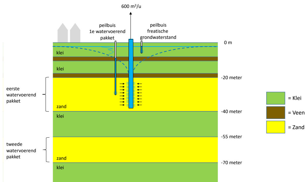
Figuur 7 Schematische weergave van onttrekkingskegel. De peilbuizen in het eerste watervoerend pakket hebben hun filter op zo'n 25 meter beneden maaiveld.
