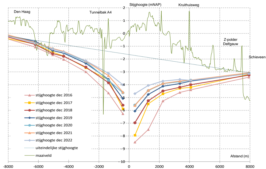
Figuur 9 Raai van noordwest naar zuidoost en de stijghoogte in het eerste watervoerend pakket.
