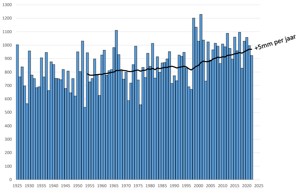
Figuur 21 Neerslag per jaar in Delft sinds 1925 ( bron: KNMI dag waarnemingen station 449 Delft)
