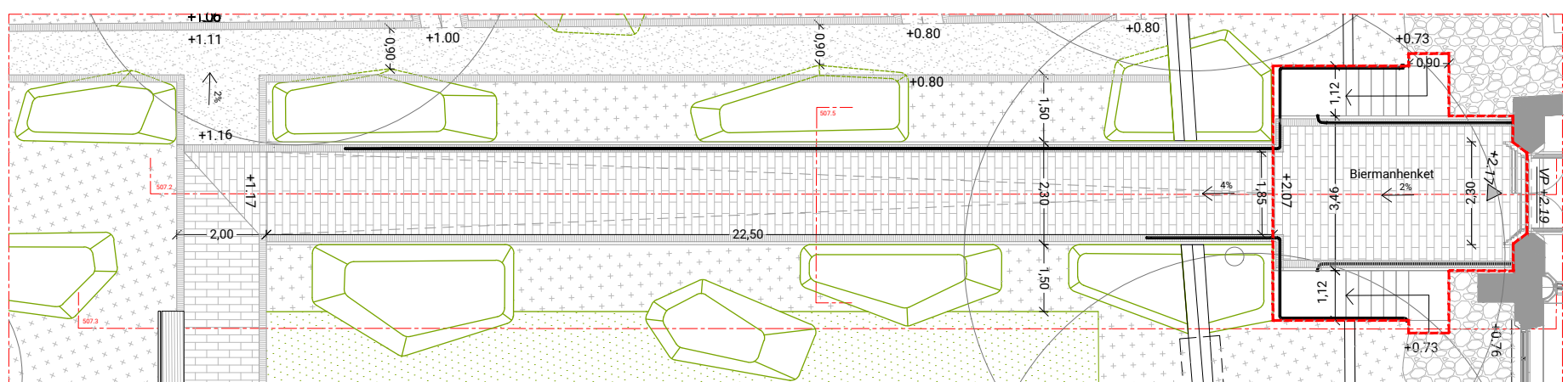
507.1 | Plan helling en bordes 1:100
