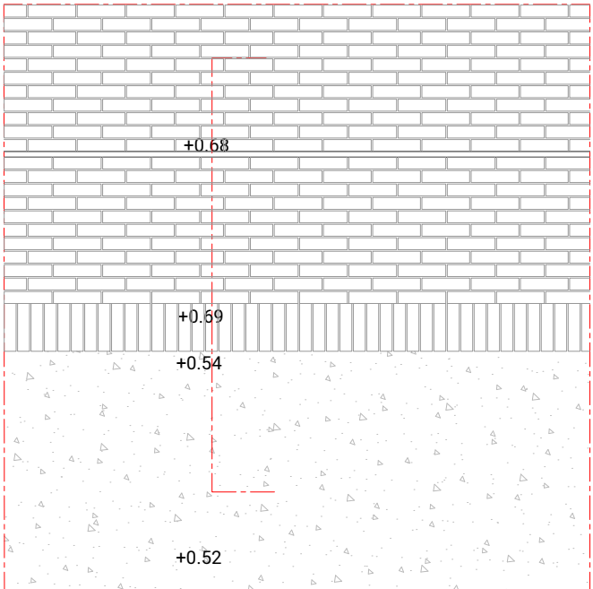
503.2 | Doorsnede inpassing sleufgoot en muur terras 1:20
