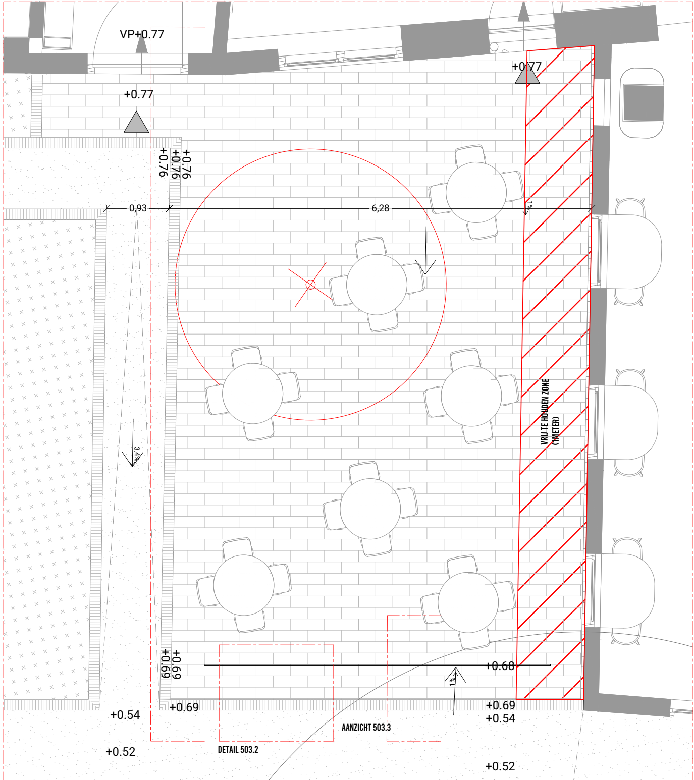
503.1 | Plattegrond terras 1:50
