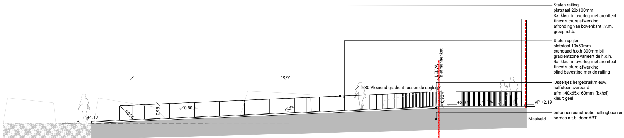
507.2 | Railing helling linkerzijde 1:100
