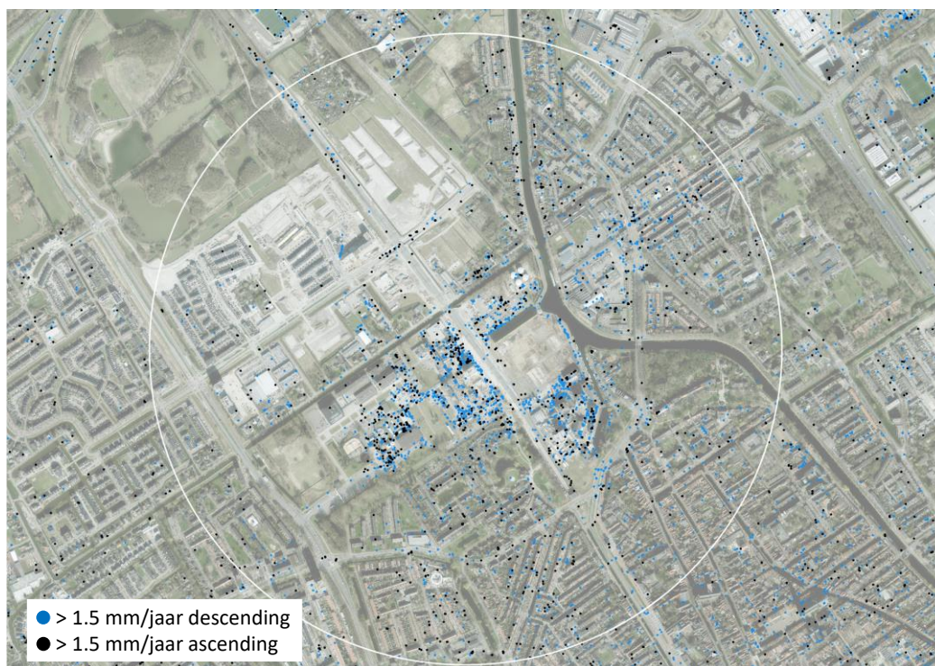
Figuur 31 Locaties in de omgeving van Delft waar het maaiveld de afgelopen 2 jaar met meer dan 1.5 mm per jaar is gestegen. De zwarte punten zijn van de opgaande baan van de TerraSAR-X satelliet en de blauwe punten van de neergaande baan.
