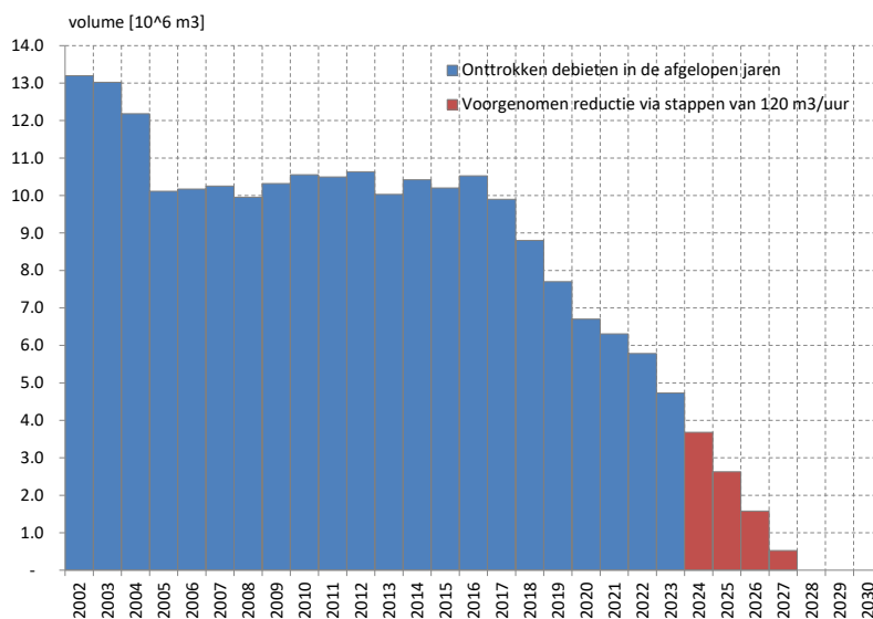
Figuur 5 Onttrokken debieten van 2002 tot en met 2023 en het voorgenomen afbouwschema waarbij de onttrekking met stappen van 120 m³/uur wordt afgebouwd.
